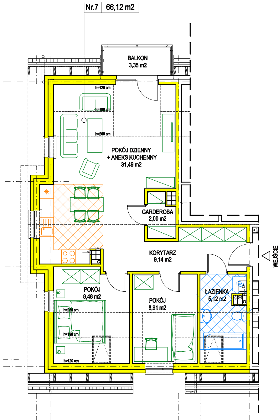
PODDASZE - rzut mieszkania D7 1:100
